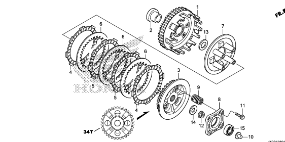
CLUTCH(2)(F.C.C.)
